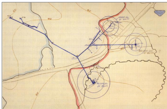
De positie van de tunnels en mijnkamers aan Kruisstraat
